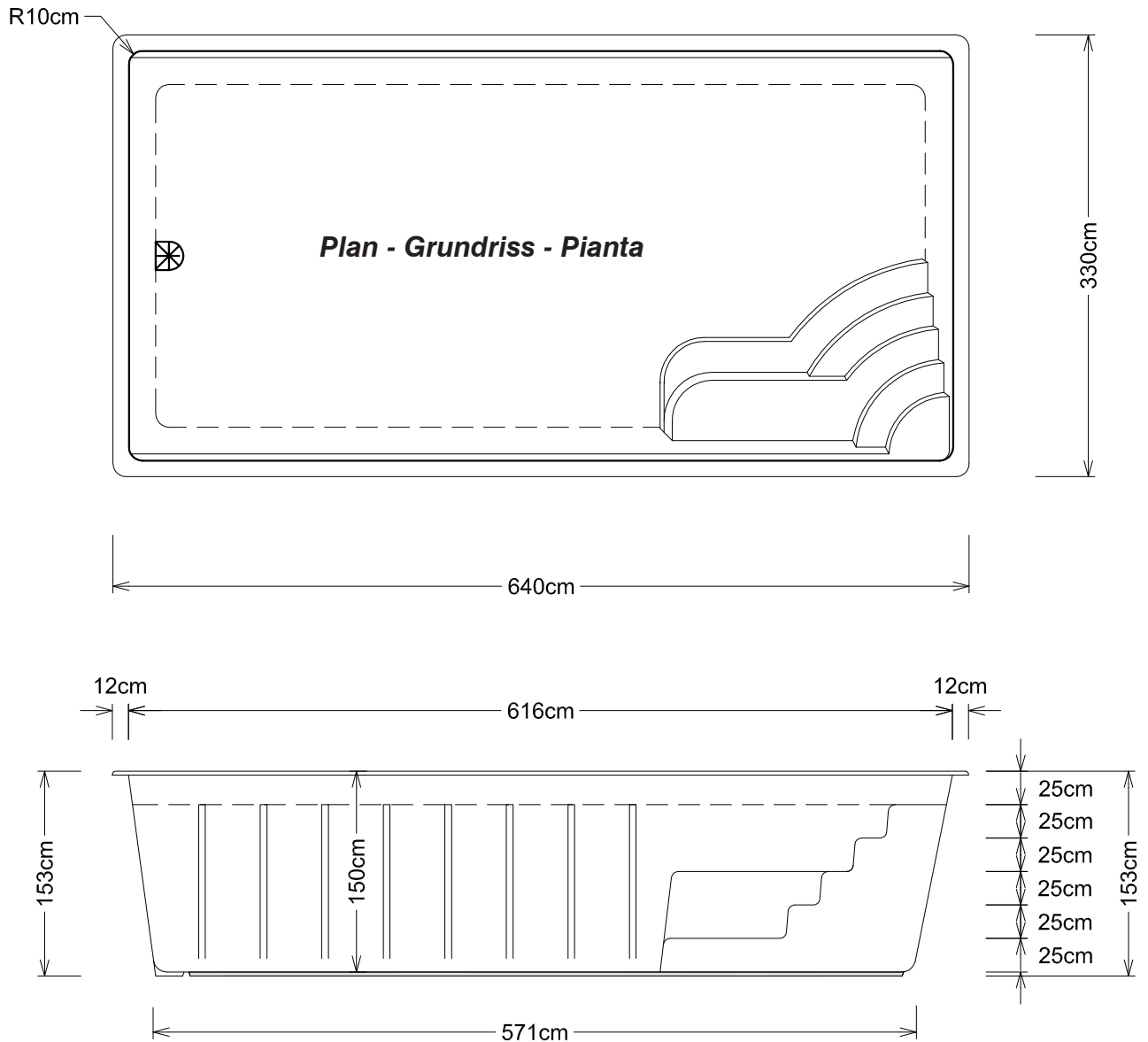
Coupe latérale - Seitenansicht - Prospetto laterale
