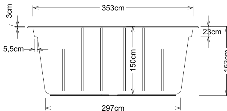
Vue coupe skimmer - Ansicht Skimmerseite - Prospetto parte Skimmer
