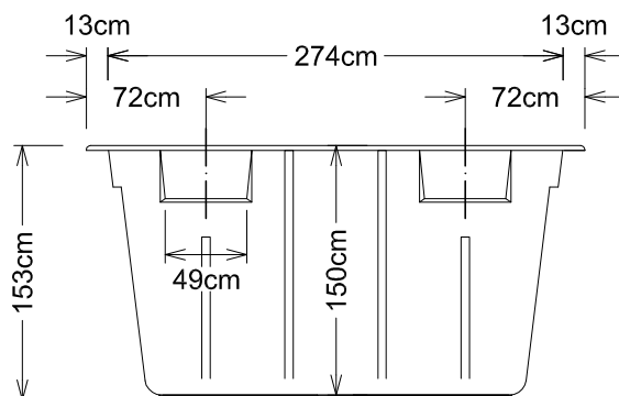
Vue coupe skimmer - Ansicht Skimmerseite - Prospetto parte Skimmer
